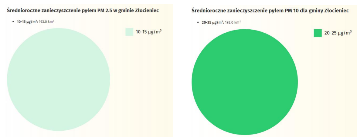
Schemat 3 Średnioroczne zanieczyszczenie powietrza w gminie Złocieniec
